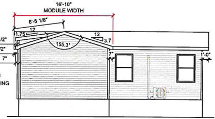
RIGHT ELEVATION
